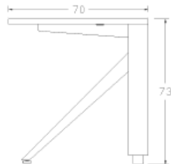
MESAS CONFERENCIAS
