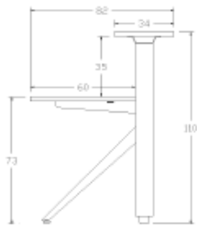
MOSTRADOR
