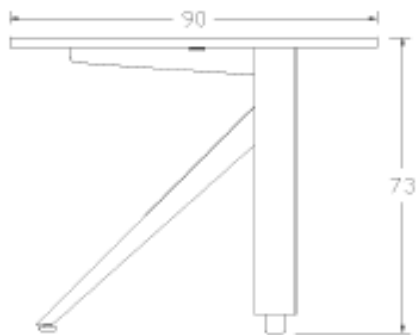
MÓDULO DISCAPACITADOS
